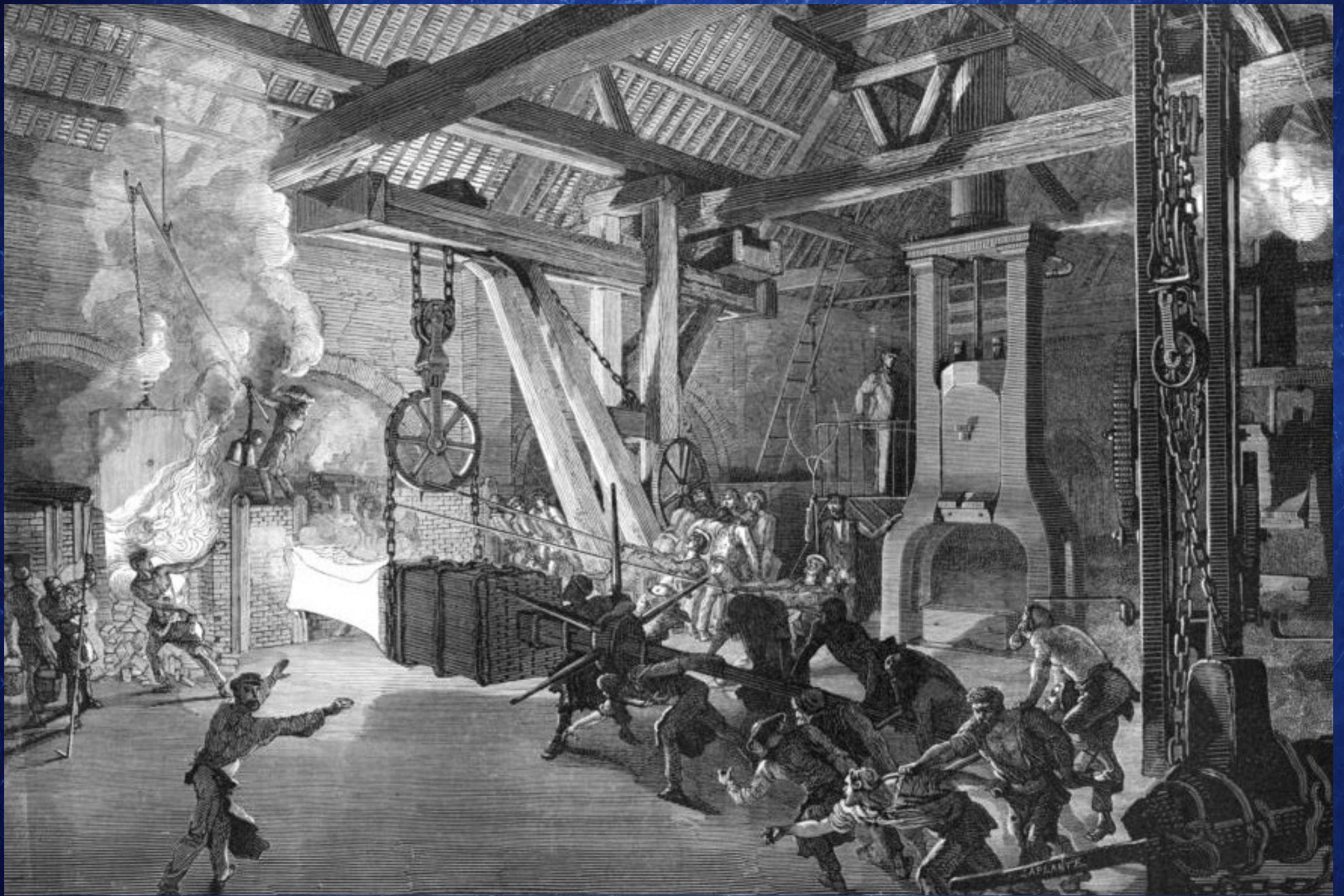
Le marteau-pilon à la forge de grosses œuvres. Les hommes manoeuvrent l'énorme pièce à la sortie du four pour la glisser sous le pilon.
